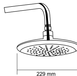
RS 0105 9" Round FCP M.R.P.: 2652.00
